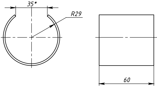
Поз.2 (Прокладка)
