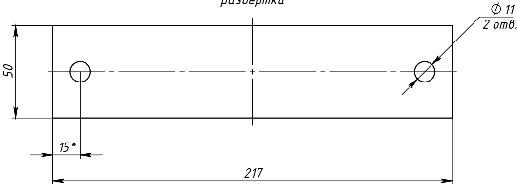
Поз.1 (Полухомут) развертка
